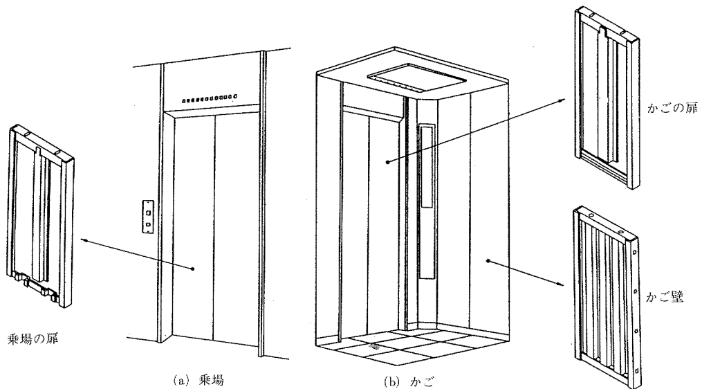
図7.1 エレベーターの意匠パネルの種類と構造
