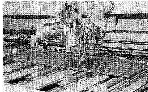
図7.3 接着剤塗布ロボット
