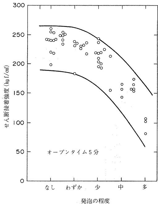
図7.7 発泡の程度とせん断接着強度
