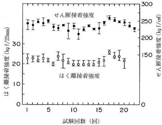
図7.4 塩ビ化粧鋼板（コーティング材料B）の接着強度の再現性
