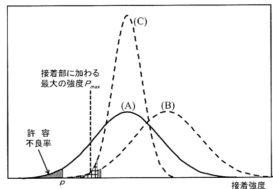
図1 不良率を低減するための二つの改善方法
