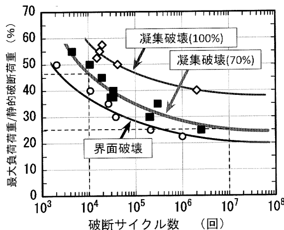
図5 凝集破壊率と疲労試験結果
